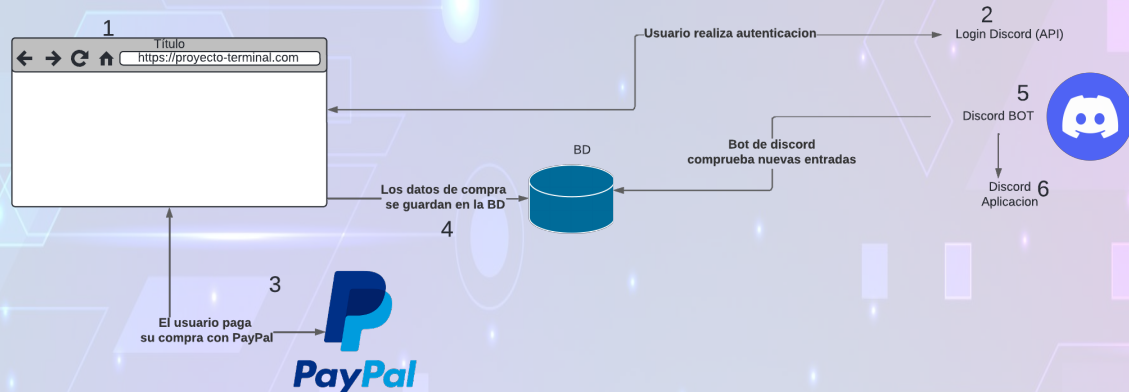
Figure 10: Diagrama general del sistema
