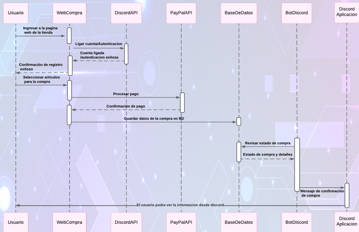
Figure 11: Diagrama secuencial del sistema
